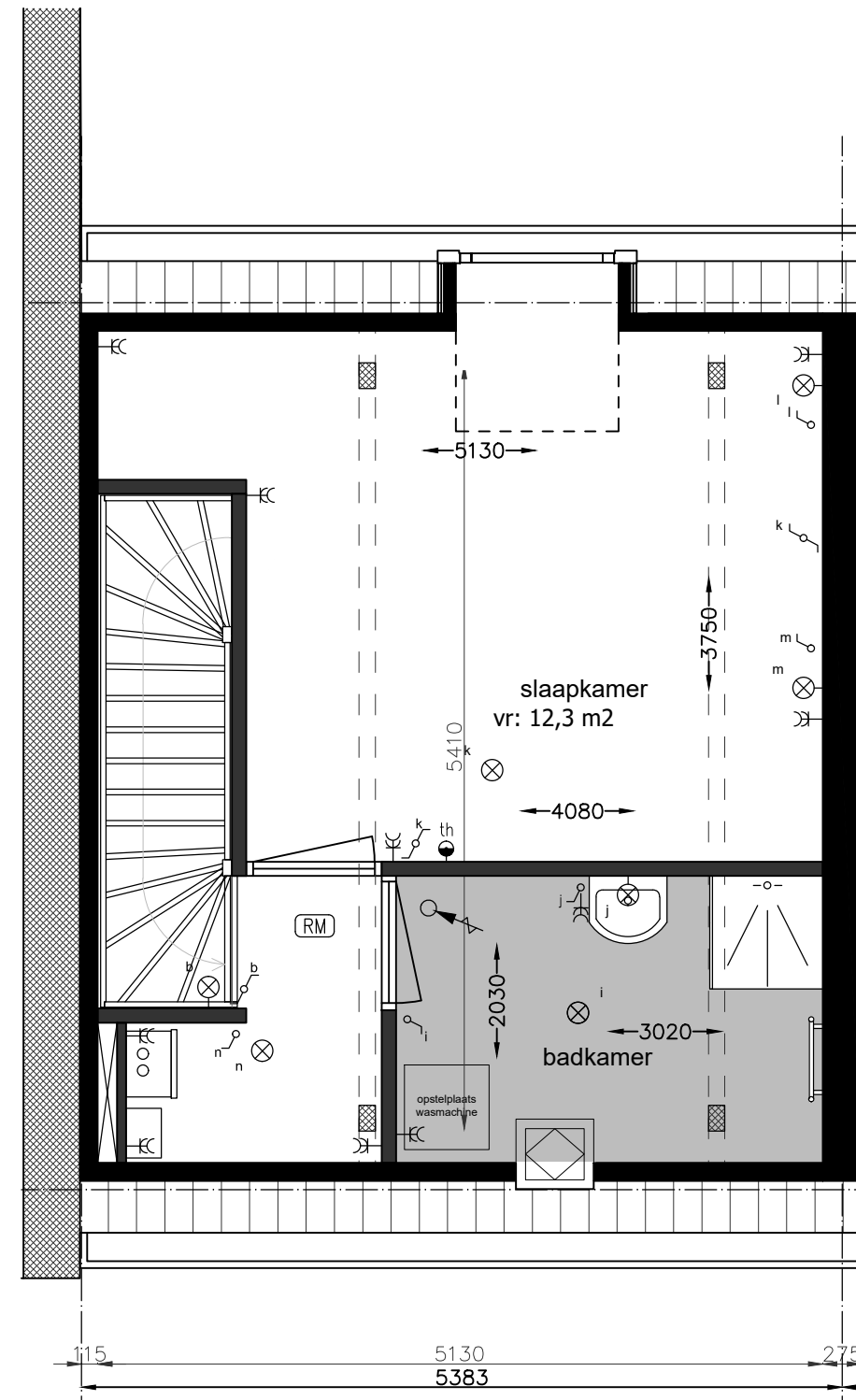
1e Verdieping ↙ 1:50
