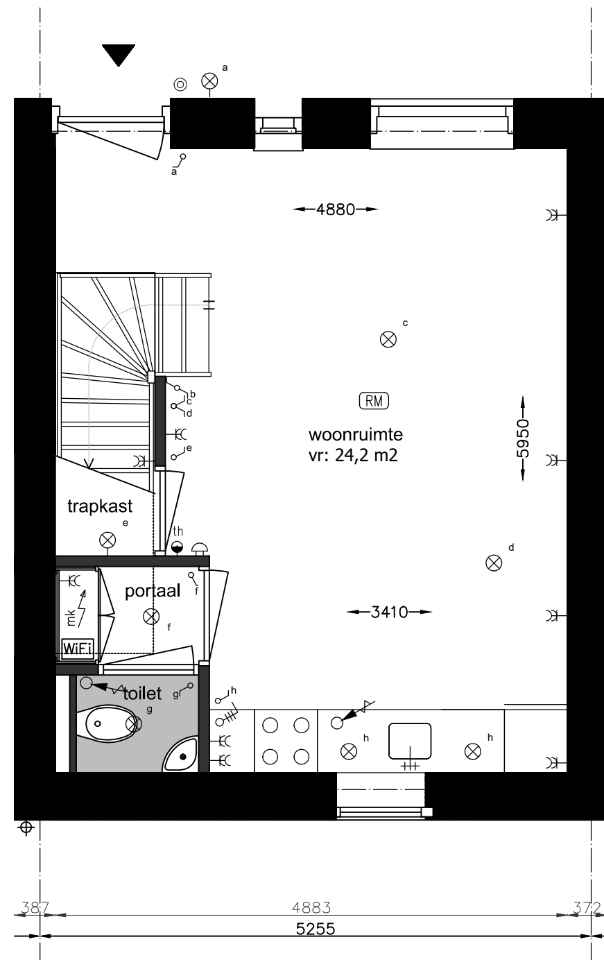
Begane Grond ↻ 1:50
