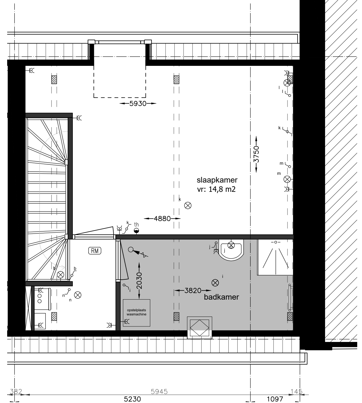
1e Verdieping ↙ 1:50
